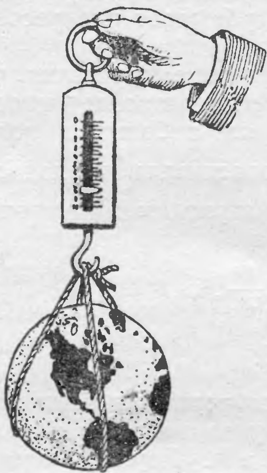
Рис. 91. На каких весах могли взвесить Землю?
