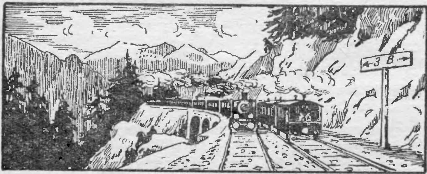
Рис. 12. Задача о двух поездах.
