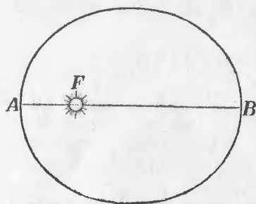
Рис. 19. Какой формы была бы орбита Земли, если бы эксцентриситет земной орбиты был равен 0,5. В фокусе F — Солнце.
