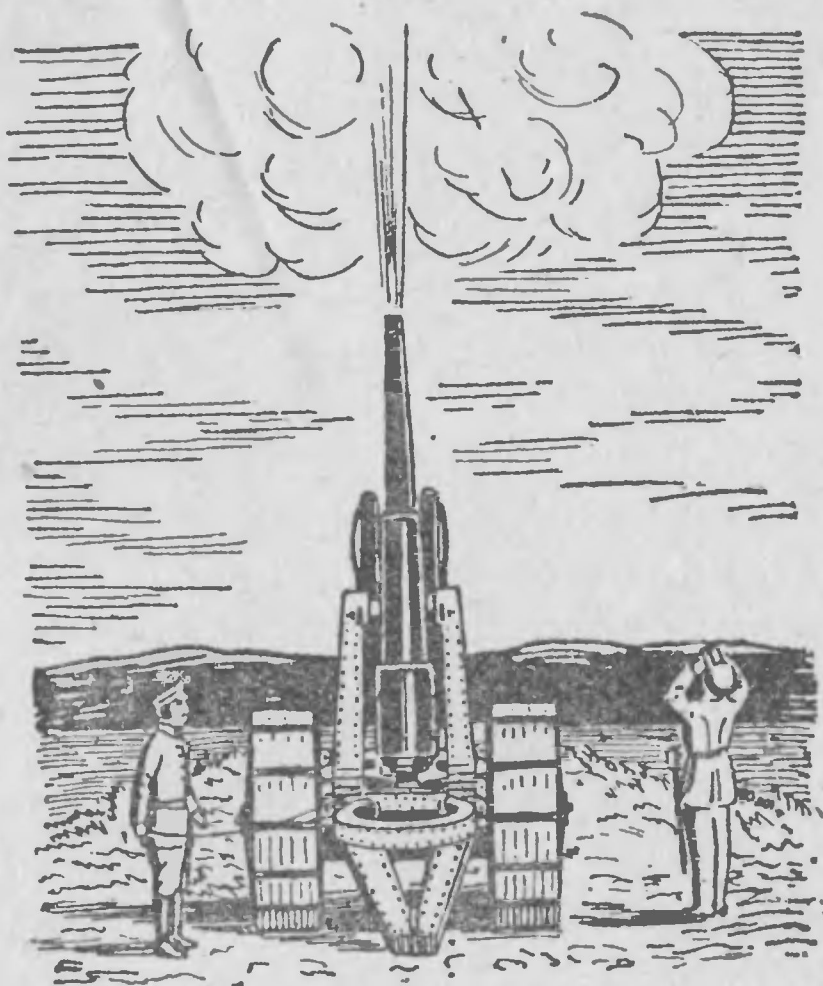
Рис. 86. Задача о пушечном ядре, брошенном отвесно.
