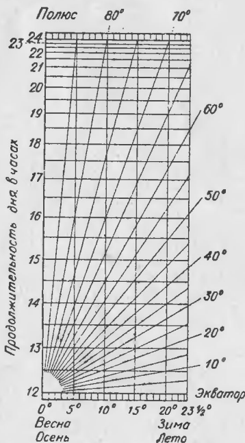
Рис. 8. Чертёж для графического определения продолжительности дня. (Объяснение в тексте.)
