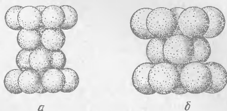
Рис. 3. Пространственная картина, показывающая два способа плотной упаковки шаров
