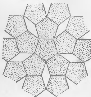
Рис. 7. С помощью правильных пятиугольников невозможно заполнить всю плоскость без просветов
