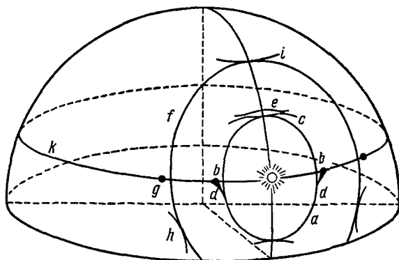
Рис. 134. Схематическое изображение некоторых наиболее важных явлений гало.
