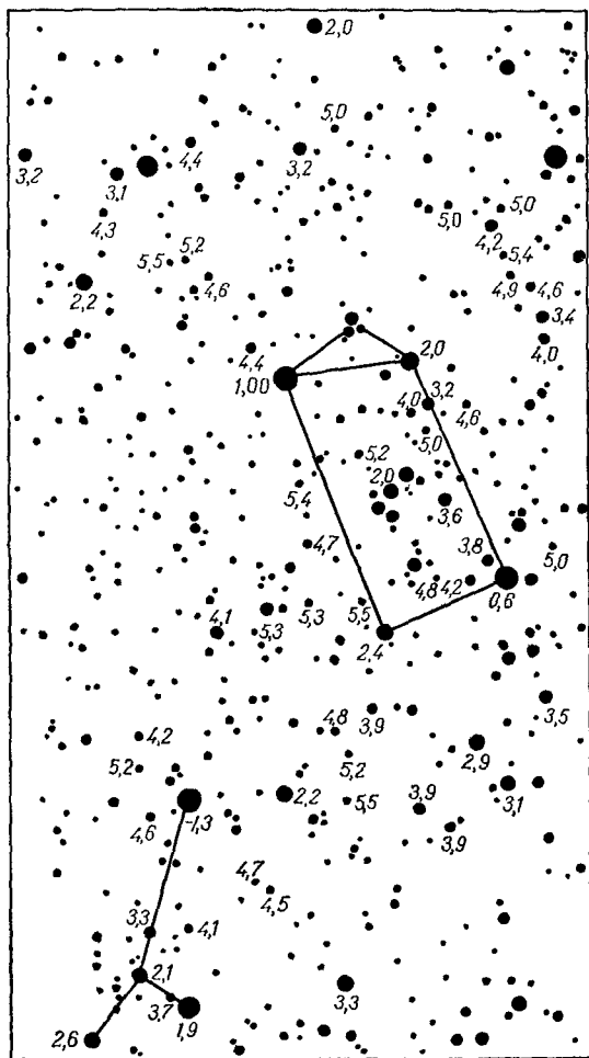
Рис. 72. Область созвездия Орiona. Числа указывают блеск звезд.
