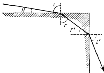
Рис. 140. Преломление светового луча прямоугольной ледяной призмой.
