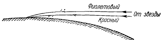
Рис. 70. Возникновение окраски при мерцании звезд.
