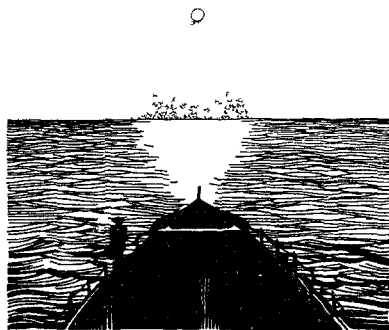
Рис. 104. Контрастный треугольник.
