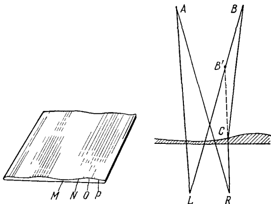
Рис. 108. Земля кажется волнистой, если смотреть на нее сквозь стекло непостоянной толщины.
