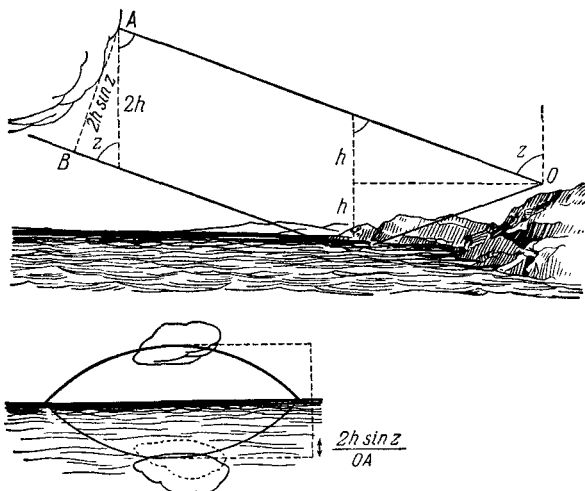
Рис. 130. Отраженная радуга.
