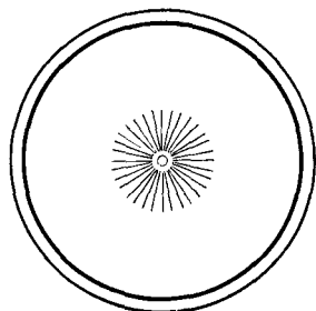
Рис. 98. Вот как выглядит быстро вращающееся велосипедное колесо.
