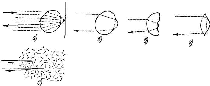
Рис. 149. Нимбы на росистой траве.
