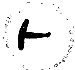
Рис 148 Глория наблюдаемая вокруг самолета.
