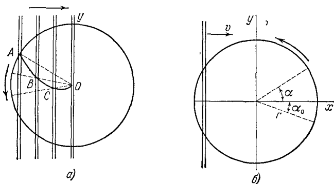
Рис. 96. Эффект «частотокола».
