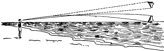
Рис. 54. Верхний мираж.
