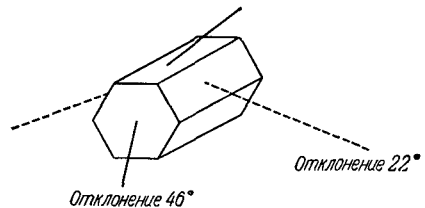
Рис. 139. В шестигранной призме угол наименьшего отклонения световых лучей может составлять или 22°, или 46°.
