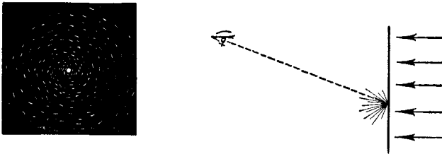
Рис. 146. Дифракция света на мелких царапинах оконного стекла.
