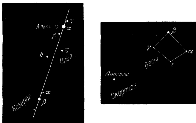
Рис. 89. Другие двойные звезды.
