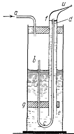
Рис. 121. Пульверизатор Автолика.
