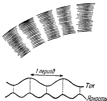
Рис. 97. Обнаружение быстрого мерцания света электрических ламп.
