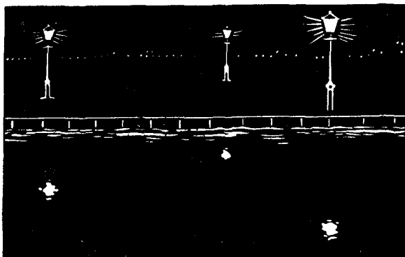
Рис. 7. Отражение может отличаться от самого предмета!
