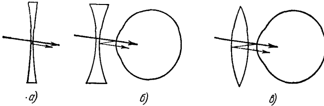
Рис. 86. Как возникает двойное отражение, если смотреть сквозь очки: а) слабые стекла; б) вогнутые стекла сильнее -5 ; в) выпуклые стекла сильнее +3 .
