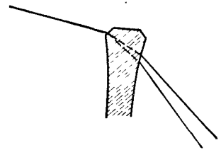
Рис. 87. Как очки создают спектр.
