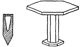
Рис. 136. Ледяные кристаллы, играющие важную роль в образовании ложных солнц.
