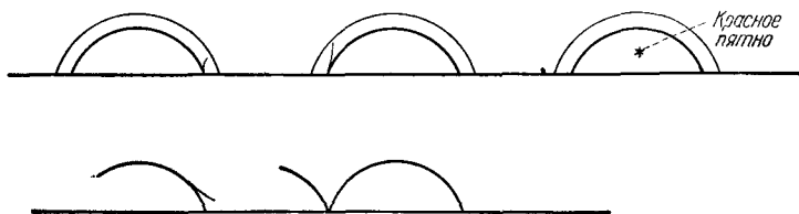
Рис. 133. Необычные радуги.
