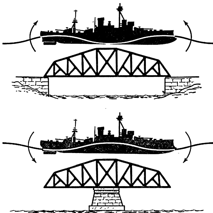
Рис. 43—44. Пароход на волнах. В обоих положениях судну угрожает поломка посередине. Почему?
