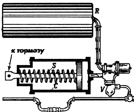
Рис. 70. Подробности устройства воздушного тормоза. Когда тормоз не работает, клапан V закрыт, и сжатый воздух из баллона R не идет в цилиндр С; пружина S оттягивает стержень, соединенный с тормозной колодкой
