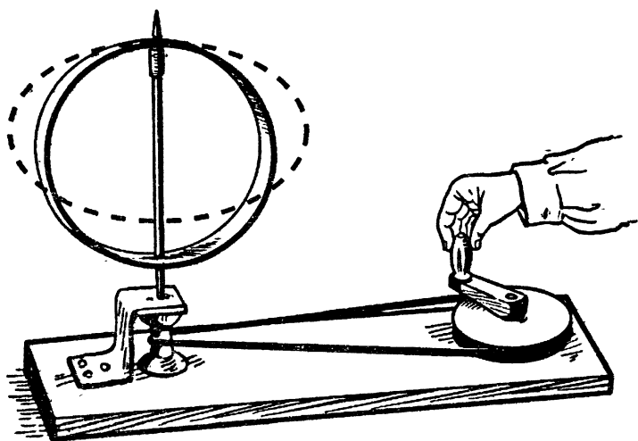
Рис. 30. Самодельная центробежная машина
