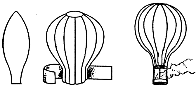
Рис. 81. Как изготавливается маленький воздушный шар из папиросной бумаги. Гондолой служит крышка от жестянки; в нее кладут смоченную спиртом ватку и поджигают; шар пускают, едва только пламя погаснет (но не ранее — иначе возможен пожар)
