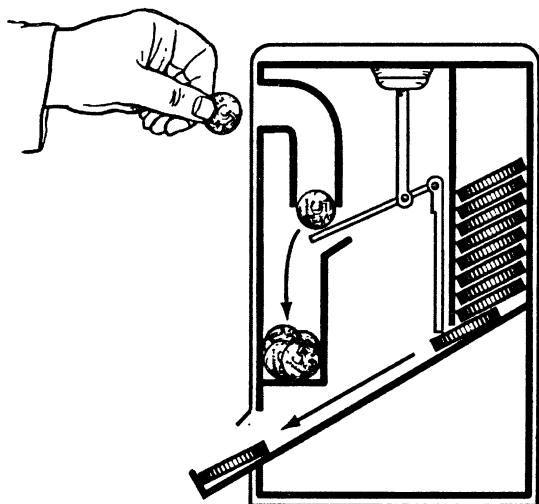
Рис. 15. Устройство билетного автомата
