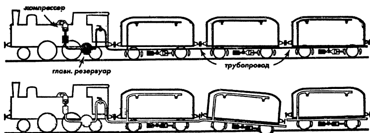
Рис. 69. Устройство воздушного тормоза для остановки поездов. Внизу показано, как действует тормоз в случае разрыва поезда. На обоих рисунках зачернены части, заполненные сжатым воздухом
