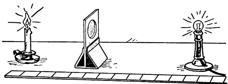
Рис. 86. Второй способ измерить силу света
