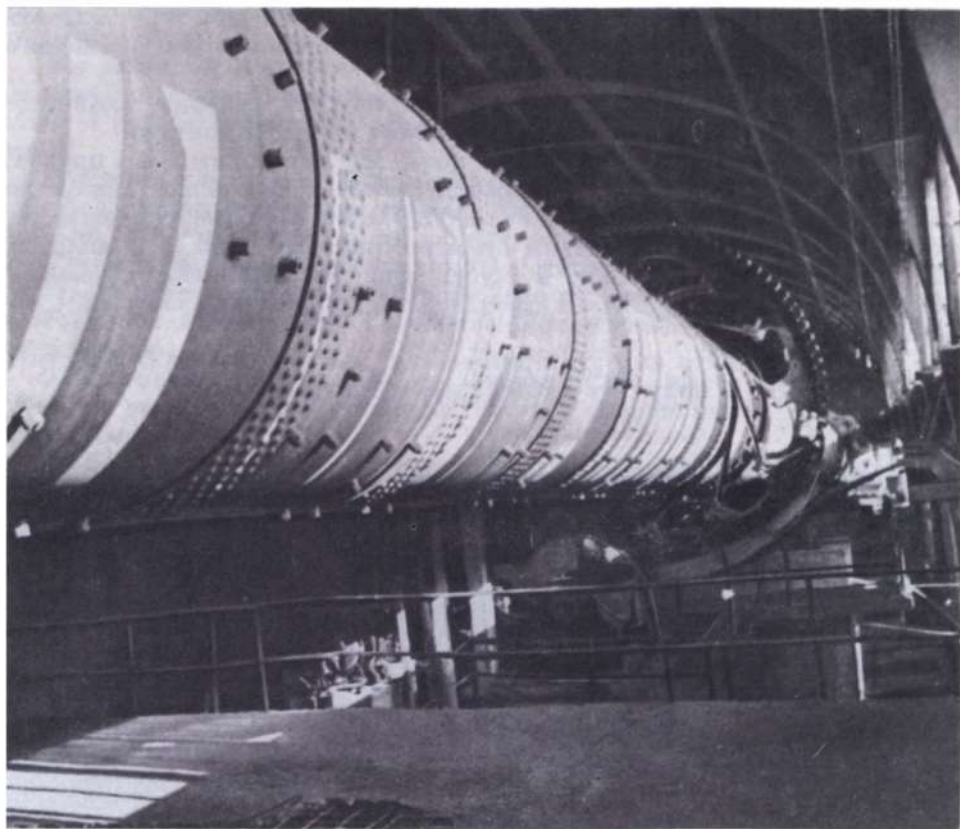
Огромная вращающаяся печь для обжига нефелина.
