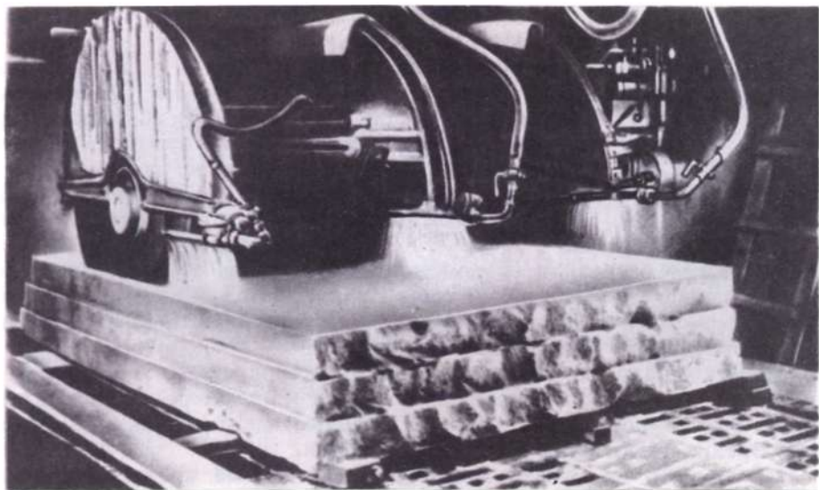
Мрамор распиливают с помощью круглых вращающихся пил, смоченных водой с порошком кварца, гранита или карборунда.
