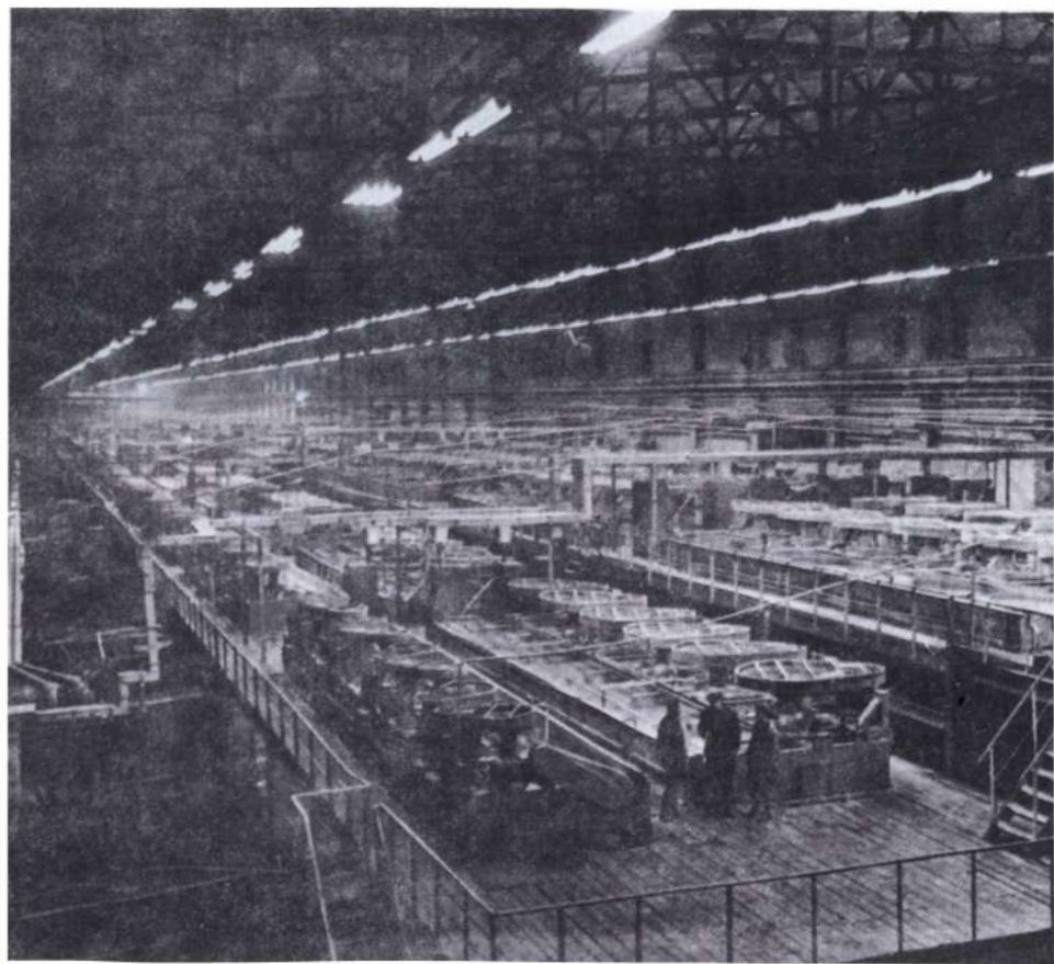
Мельнично-флотационный цех апатито-нефелиновой обогатительной фабрики. Мурманская область.
