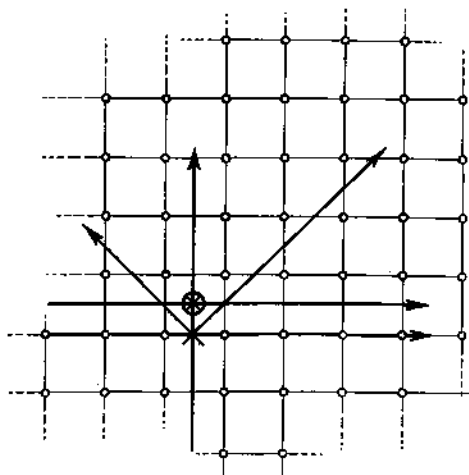
Кристаллическая решетка на плоскости.
