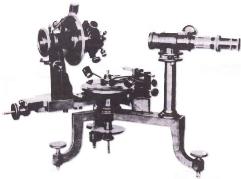
Гониометр — прибор для измерения углов кристаллов, сконструированный русским кристаллографом академиком Е. С. Федоровым.
