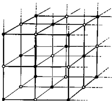
Кристаллическое строение новой соли — хлористого натрия. Черные шарики — атомы хлора, белые — атомы натрия.
