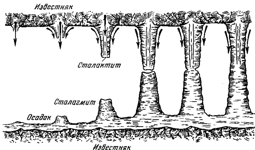
Схема, показывающая, как растут сталактиты и сталагмиты и образуются колонны.
