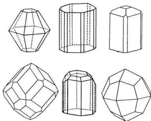
Природные формы кристаллов разных минералов: корунда, берилла, везувияна, граната, топаза, лейцита.
